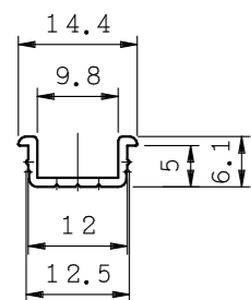
アルミロング引手 ALH12 (S=1/1)
